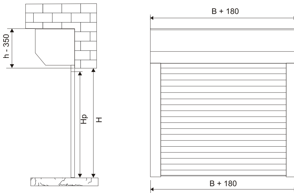
Parametry montażowe bramy ze skrzynią SK 300
