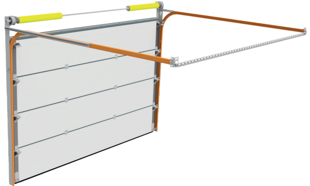
Prowadzenie S – wys. nadproża min. 350 mm
