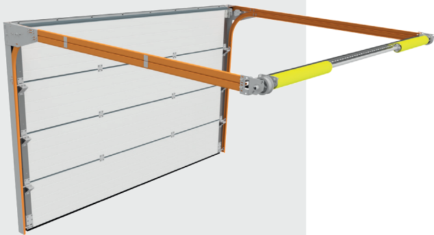
Prowadzenie R – wys. nadproża min. 80 mm (ręczna) lub 120 mm (automatyczna)
