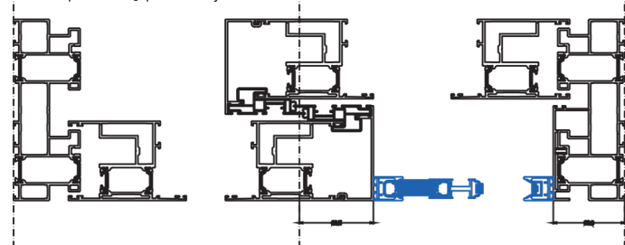
przekrój poziomy
