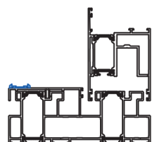
przekrój poziomy
