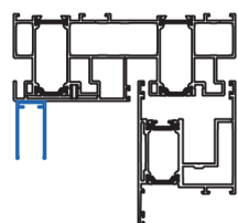
przekrój pionowy
